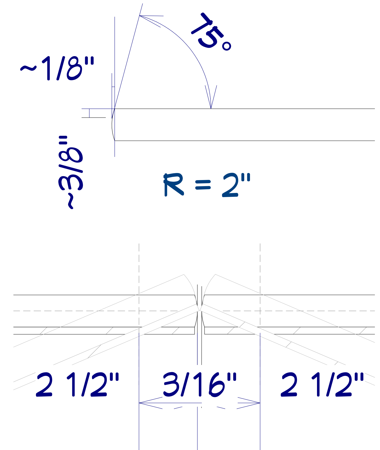
Door edge
