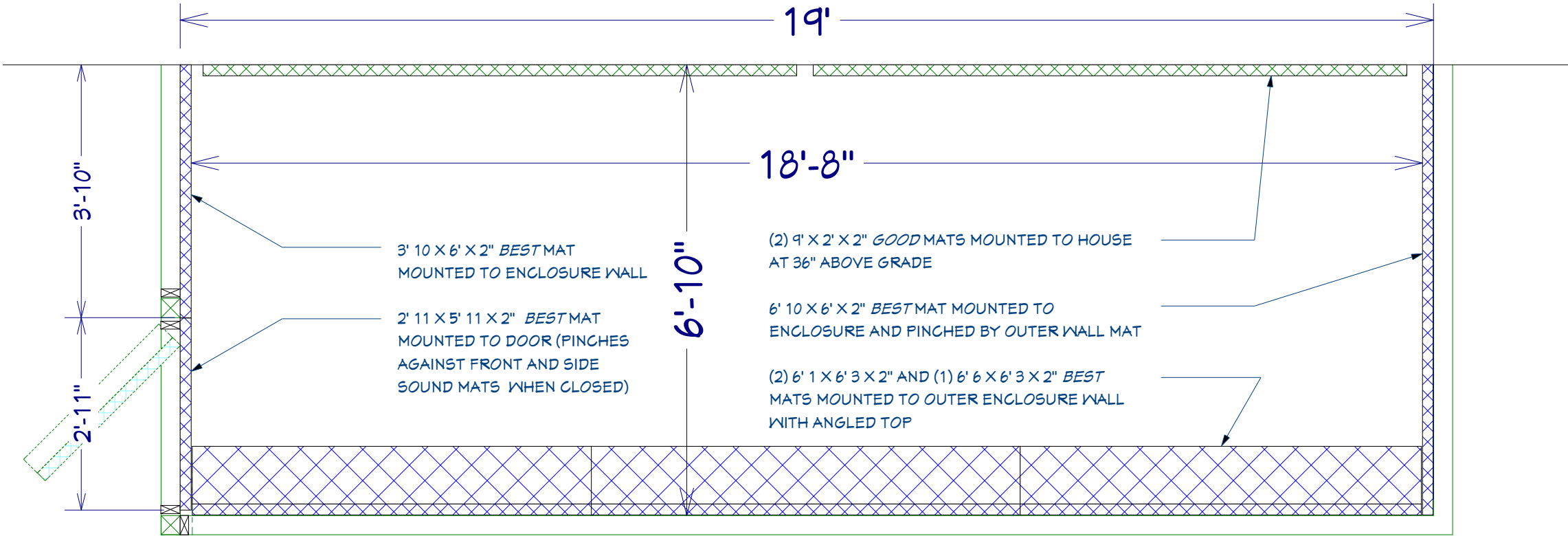
Section 1 Scale: 1" = 1'
